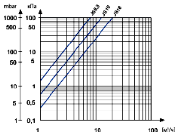
Рис.1 Графіки залежності втрати тиску лічильників від об'ємної витрати
