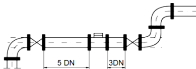
Рис. 4 Схема встановлення лічильника води
